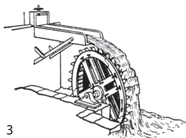
Vízikerék: 1) alulcsapott; 2) középen csapott; 3) felülcsapott.
