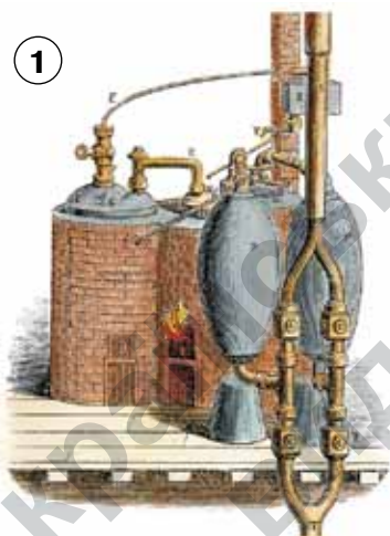
Двигун Савері, 1698
