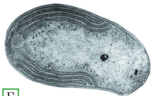
Рис. 6.4. Нітрифікатори ґрунту
