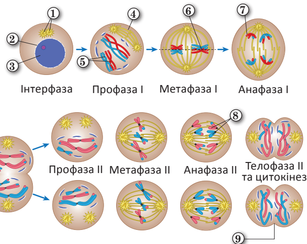
Рис. 31.4. Фази мейозу
