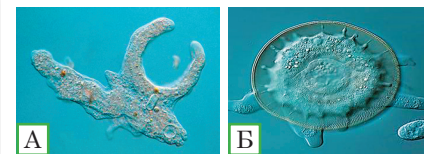
Рис. 7.10. Амебозої
