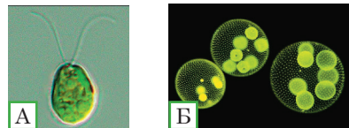
Рис. 7.8. Зелені водорості
