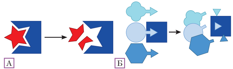
Рис. 17.3. Специфічність ферментів
