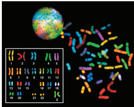
Рис. 30.4. Каріотип людини
