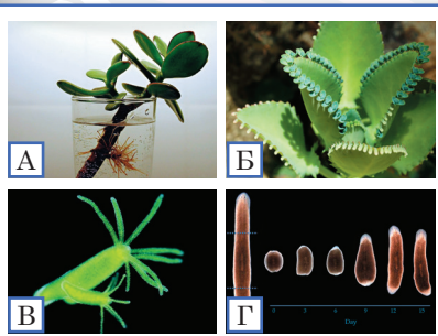
Рис. 39.1. Вегетативне розмноження
