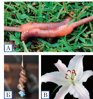
Рис. 39.3. Гермафродити
