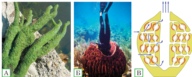
Рис. 10.1. Губки
